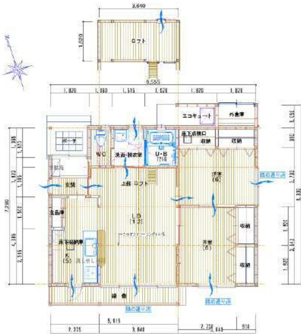
平面図 床面積=67.06㎡ (20.3坪) (外倉庫除)
