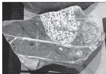
写真2 戸台層の礫岩切断研磨標本 大鹿村中央構造線博物館で展示中
