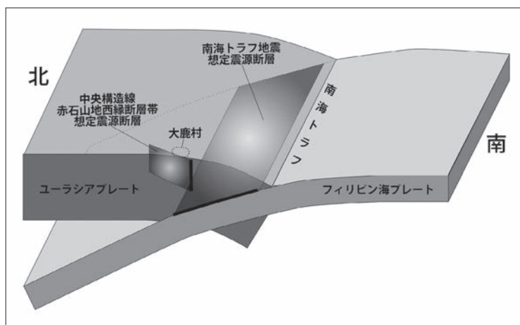
図2 南海トラフ地震と中央構造線赤石山地西縁断層帯の想定震源断層の位置関係イメージ図
