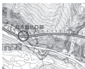
位置及びトンネル計画
