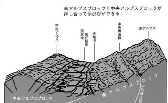
図1 中央アルプス・伊那谷・南アルプスを横切ったときの模式的な断面図 松島・岡田(1993)「伊那谷構造盆地の活断層と南アルプスの中央構造線」より引用
